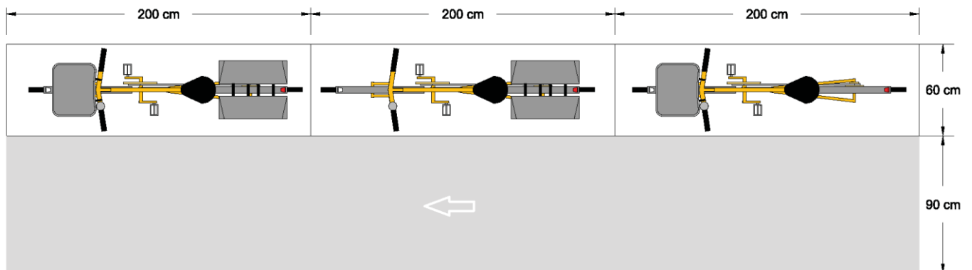
Figure 12 : Disposition longitudinale
